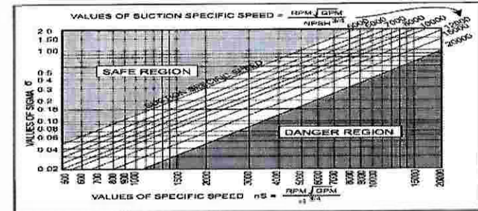
Fig. 12 Cavitation Parameter \sigma (sigma) vs. N_s & N_{ss} [20]
